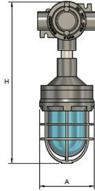
EVC-1100 EVC-2200
